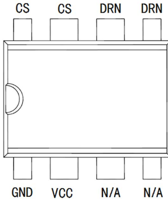
DIP8 封装
