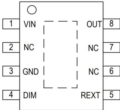
ESOP8
