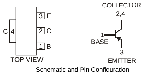
SOT89-3L
