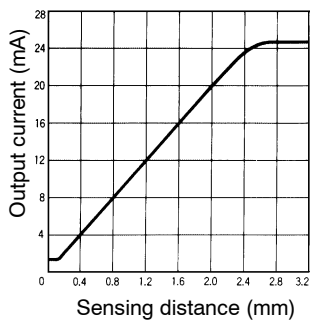
E2CA-X2A
