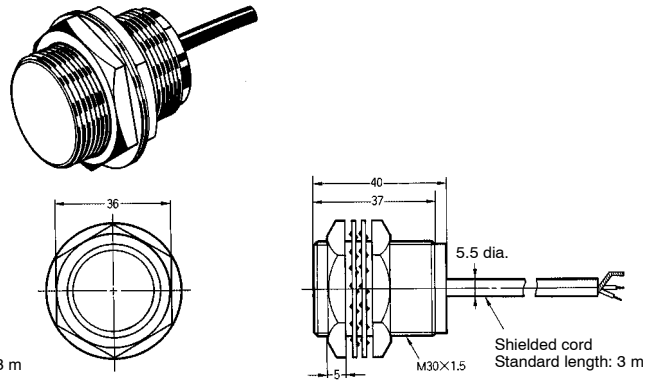
E2CA-X10A
