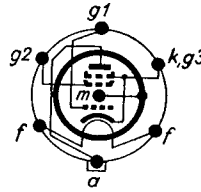
Sockelschaltenschema
