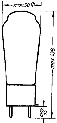
Kolbenabmessungen
