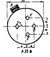
E 435 kan met bovenstaande hulzen geleverd worden.
