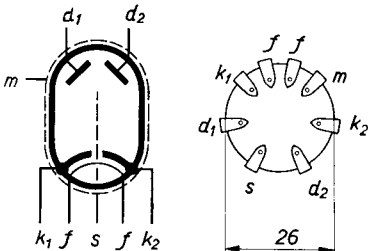
Schematische voorstelling van de duo-diodē EB 4, henevens schema van aansluiting der elektroden aan de huls.
