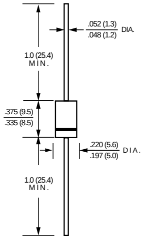
DO-201AD
