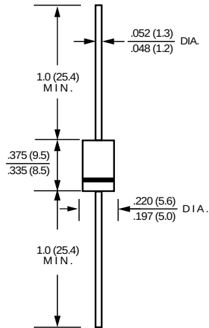
DO-201AD
