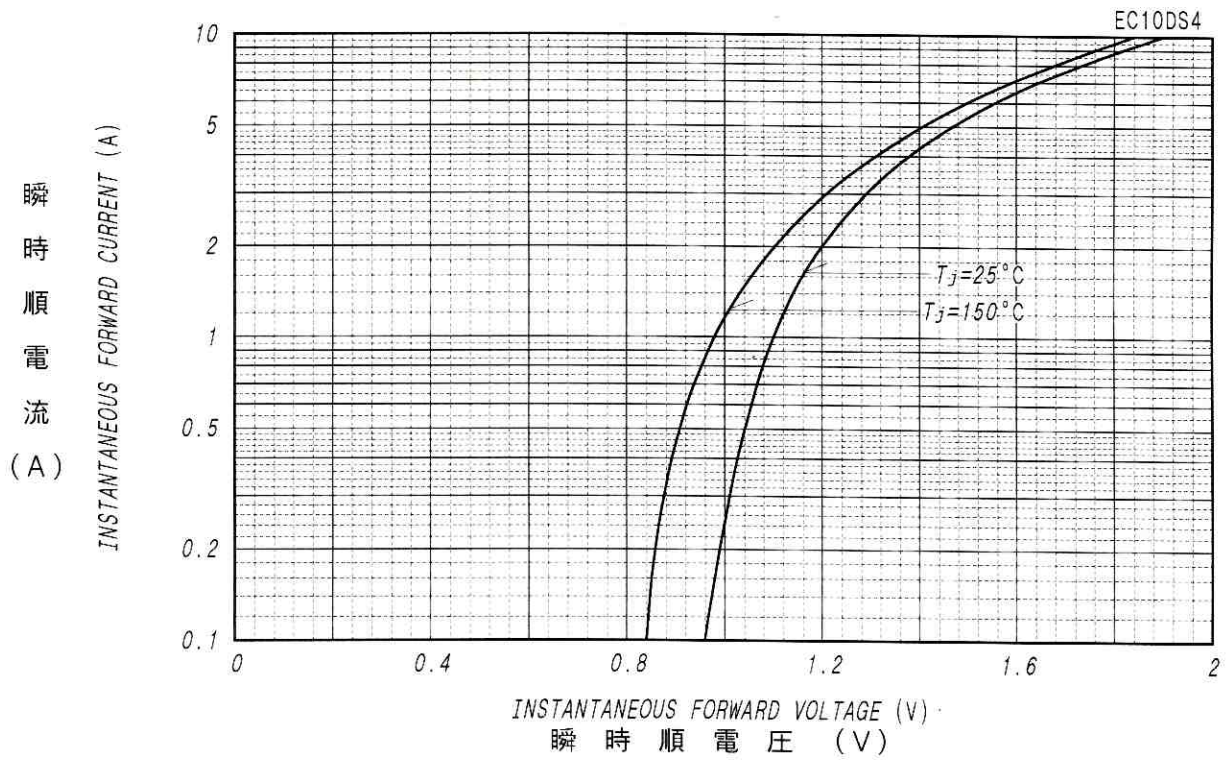
順電圧特性 FORWARD CURRENT VS. VOLTAGE
