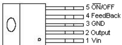
TO220B-5L/TO220-5L
