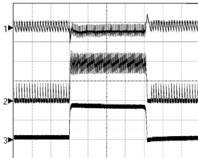
V_{OUT}=1.1V , Load Transient 1A \rightarrow 18A \rightarrow 1A
