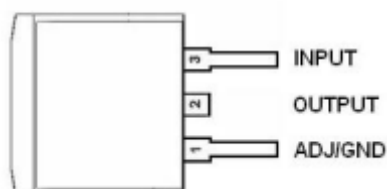
Package: TO-263-2L
