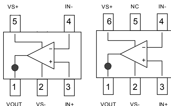
SOT25/TSOT25
