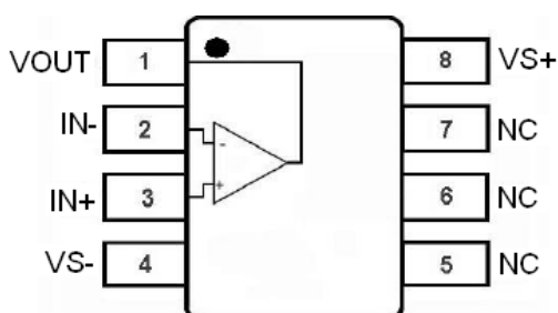
TSSOP-8
