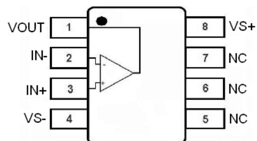
TSSOP-8
