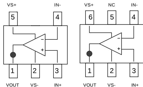
SOT25/TSOT25
