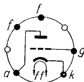
Sockelschaltenschema
