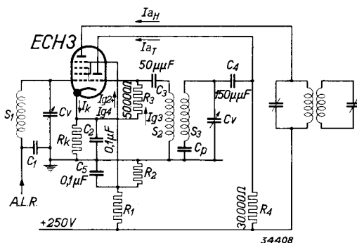
Abb. 28 Grundsätzliches Schaltbild für die Verwendung der ECH 3 als Misch- röhre. Für den Kondensator C_4 kann unter Umständen ein Wert von 100 \mu\text{F} eine im Wellenbereich gleichmäßigere Oszillatorspannung erhalten werden.
