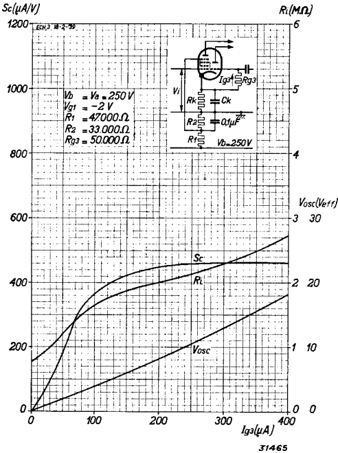
Mischteilheit S_c , Innenwiderstand R_i und effektive Oszillatorwechselspannung V_{osc} als Funktion des Oszillatorgitterstroms I_{g3} bei R_{g3} = 50.000 \Omega , V_a = 250 V und Schirmgitterspeisung über einen Spannungsteiler von 47.000 + 33.000 \Omega (rauscharme Einstellung).
