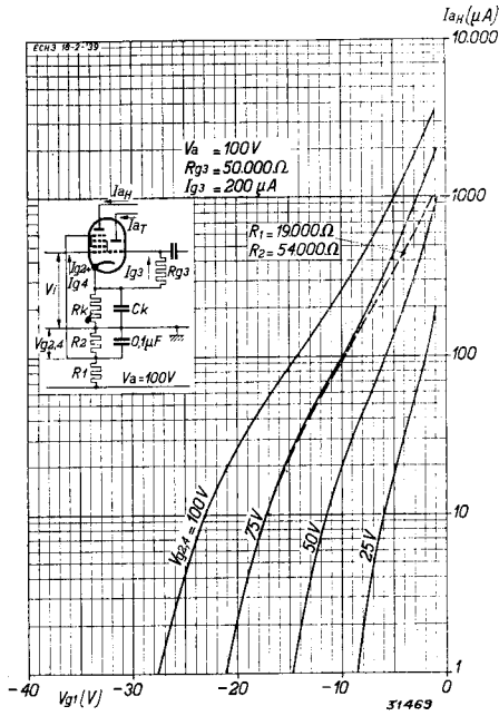
Abb. 6 Anodenstrom des Hexodenteiles als Funktion der negativen Gittervorspannung bei verschiedenen Schirmgitterspannungen und einer Anodenspannung von 100 V.
