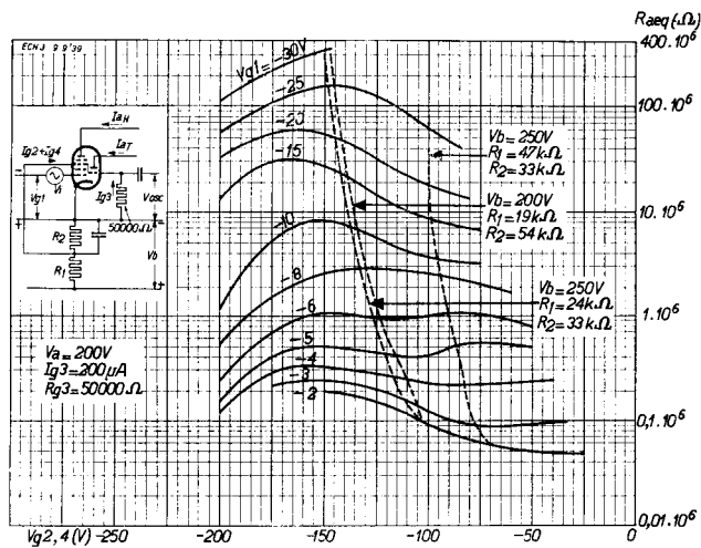
Abb. 23 Äquivalenter Rauschwiderstand R_{a_{eq}} als Funktion der Schirmgitterspannung V_{g2+4} bei verschiedenen negativen Gittervorspannungen V_{g1} .
