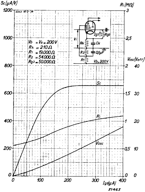
Abb. 13 Mischteilheit S_c , Innenwiderstand R_i und effektive Oszillatorwechselspannung V_{osc} als Funktion des Oszillatorgitterstroms I_{g3} bei R_{g3} = 50.000 \text{ Ohm} , V_a = 200 \text{ V} und Schirmgitterspeisung über einen Spannungsteiler von 19.000 + 54.000 \text{ Ohm} (für umschaltbare G/W-Geräte).
