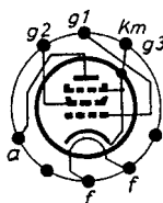
Sockelschaltchema
