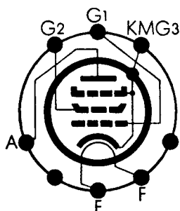
Sockelschaltbild
