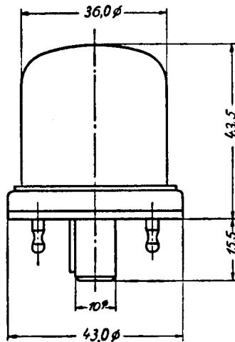
Kolbenabmessungen
