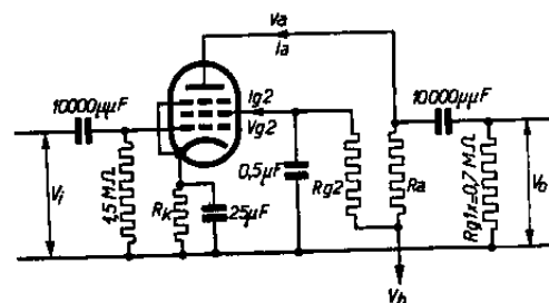
Montage de la lampe EF6 comme amplificatrice B.F. avec couplage par résistance.
