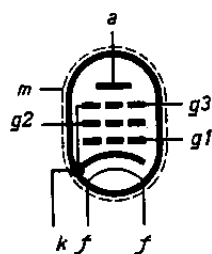
Disposition des électrodes et connexions du culot.
