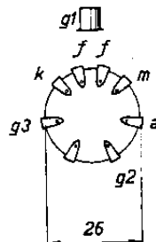
Disposition des électrodes et connexions du culot.
