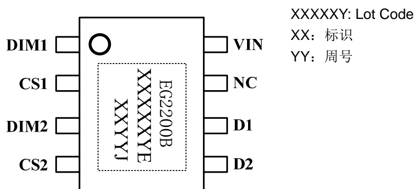
图 2 管脚封装图
