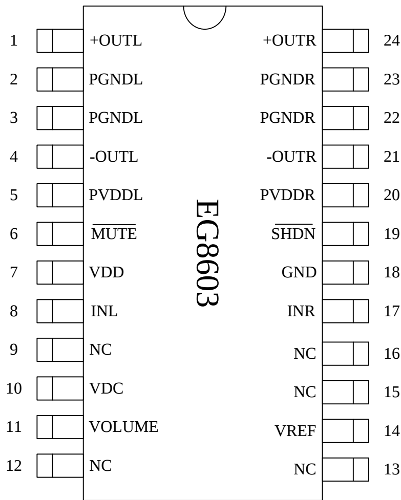
图 4-1. EG8603—SSOP24 管脚定义
