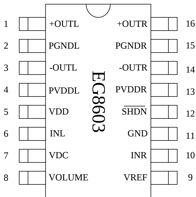
图 4-3. EG8603—SOP16 管脚定义
