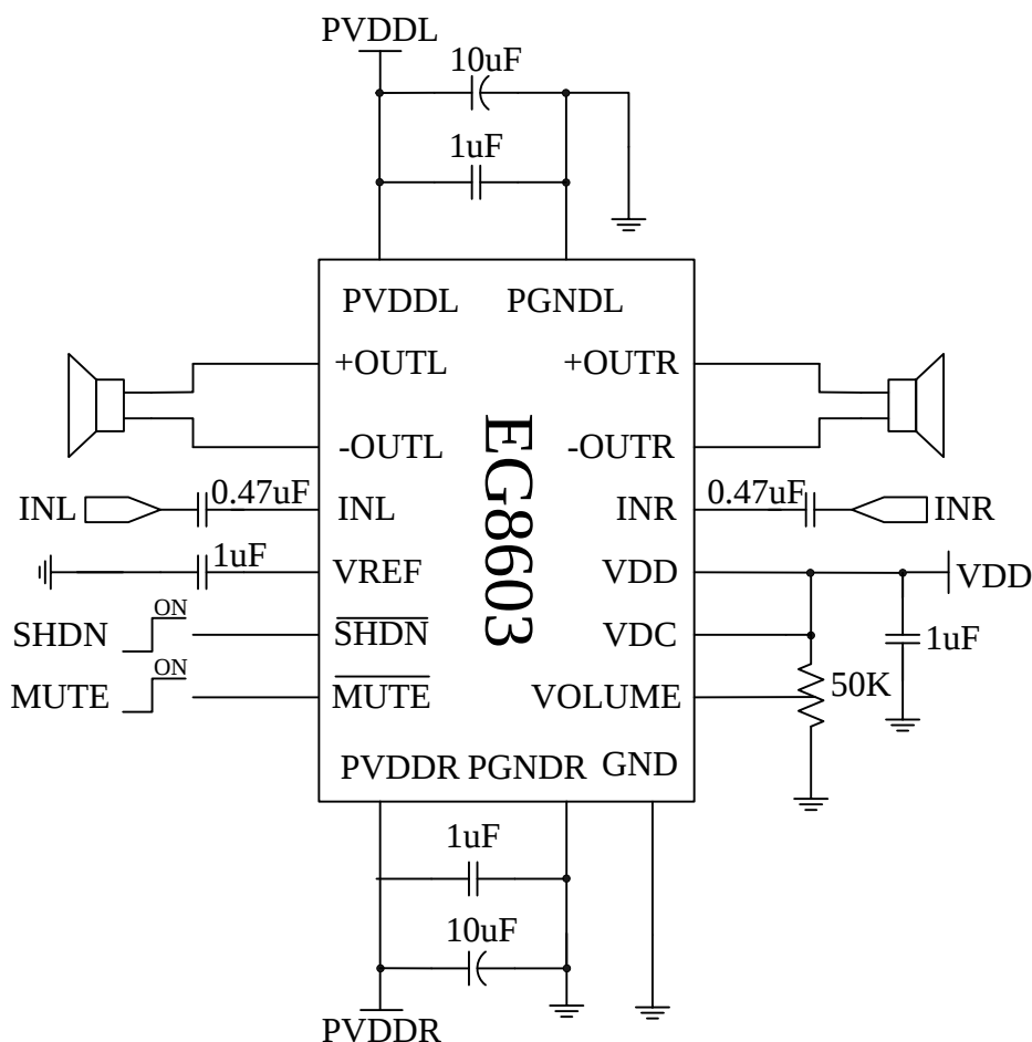
图 6-1. EG8603 典型应用电路图
