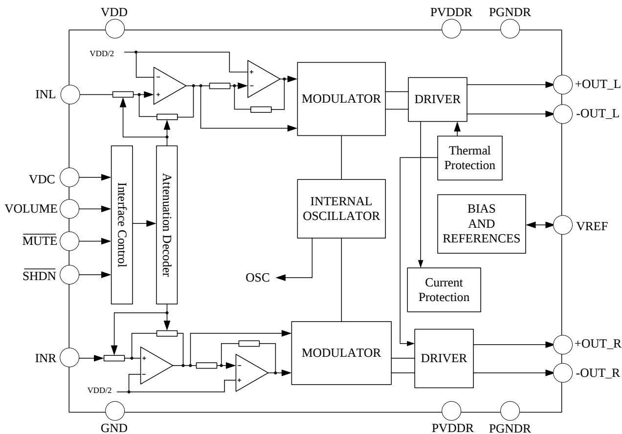
图 5-1. EG8603 结构框图
