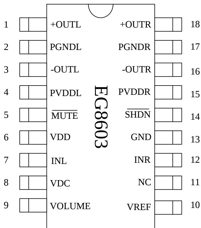
图 4-2. EG8603—SOP18 管脚定义
