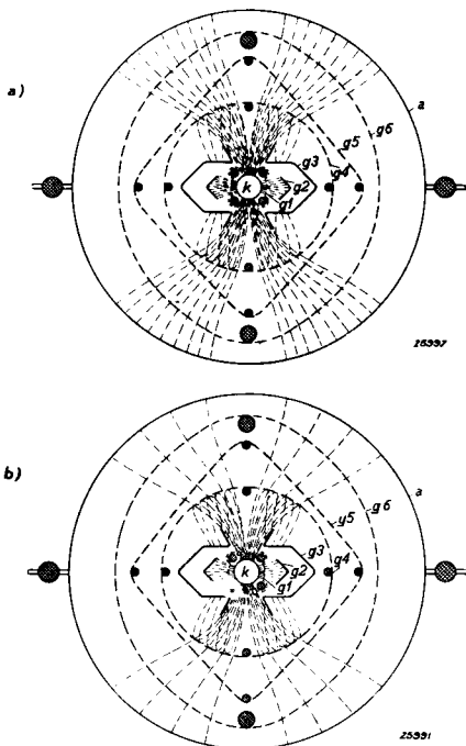
a) Doorsnede van het electroden-systeem van de EK 3, waarbij het verloop van de electronbanen is aangegeven in ongeregelde toestand. b) Dezelfde doorsnede met de electronbaenn in geregelden toestand.
