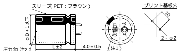
寸法図 ( CE692 形 ) [ mm ]
