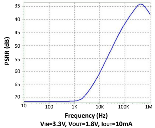
PSRR
