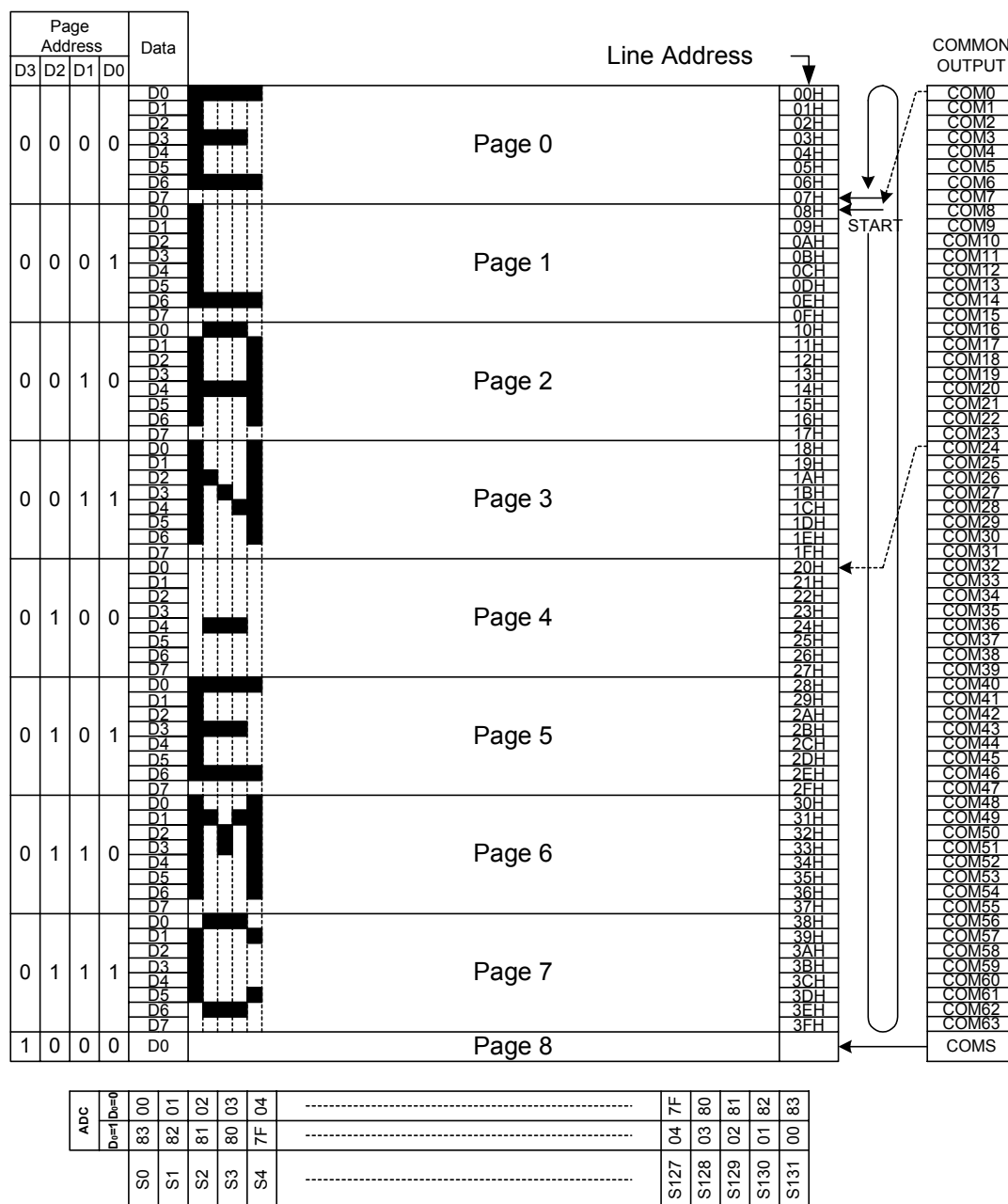
Fig. 5 Display Data RAM
