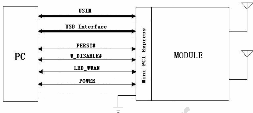
Figure 1-3 Mini PCI Express identification
