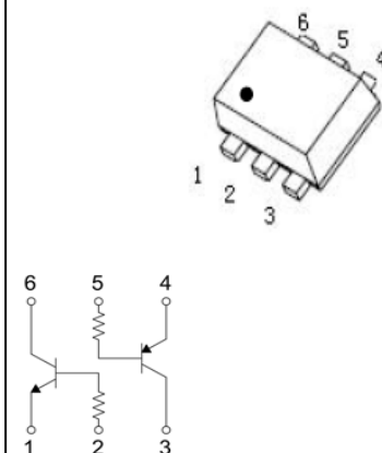
SOT-563
