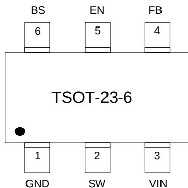
TSOT-23-6
