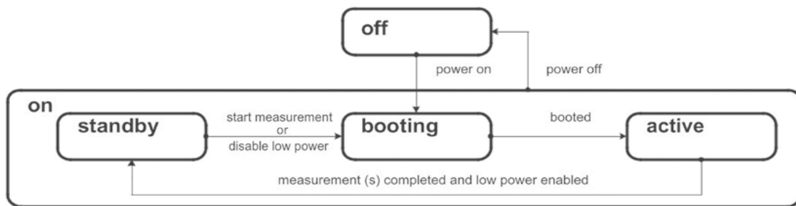
Figure 4: ENS212A power states
