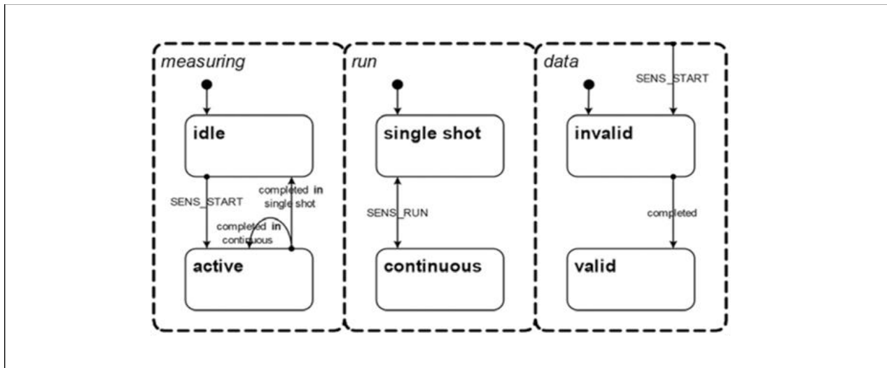
Figure 11: The ENS212A sensor modes
