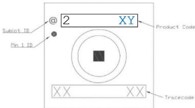
Figure 21: ENS212A marking
