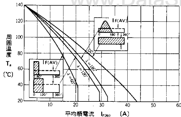
平均順電流—周囲温度 (冷却体AH01-8B) 自冷
