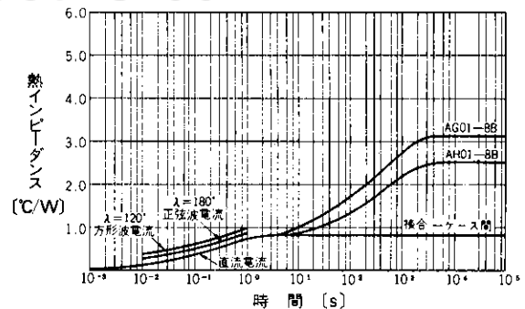
過渡熱インピーダンス(定損失)
