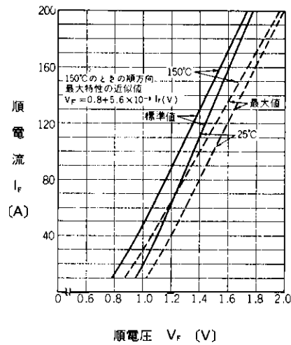
順特性
