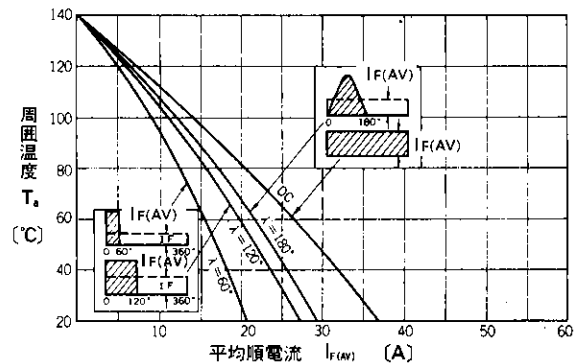
平均順電流—周囲温度 (冷却体AG01-8B) 自冷
