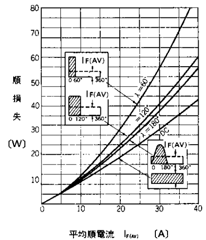
順損失
