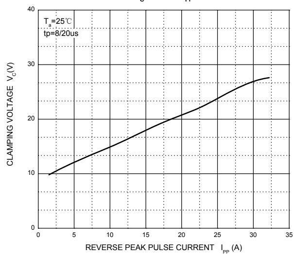
V_C — I_{PP}
