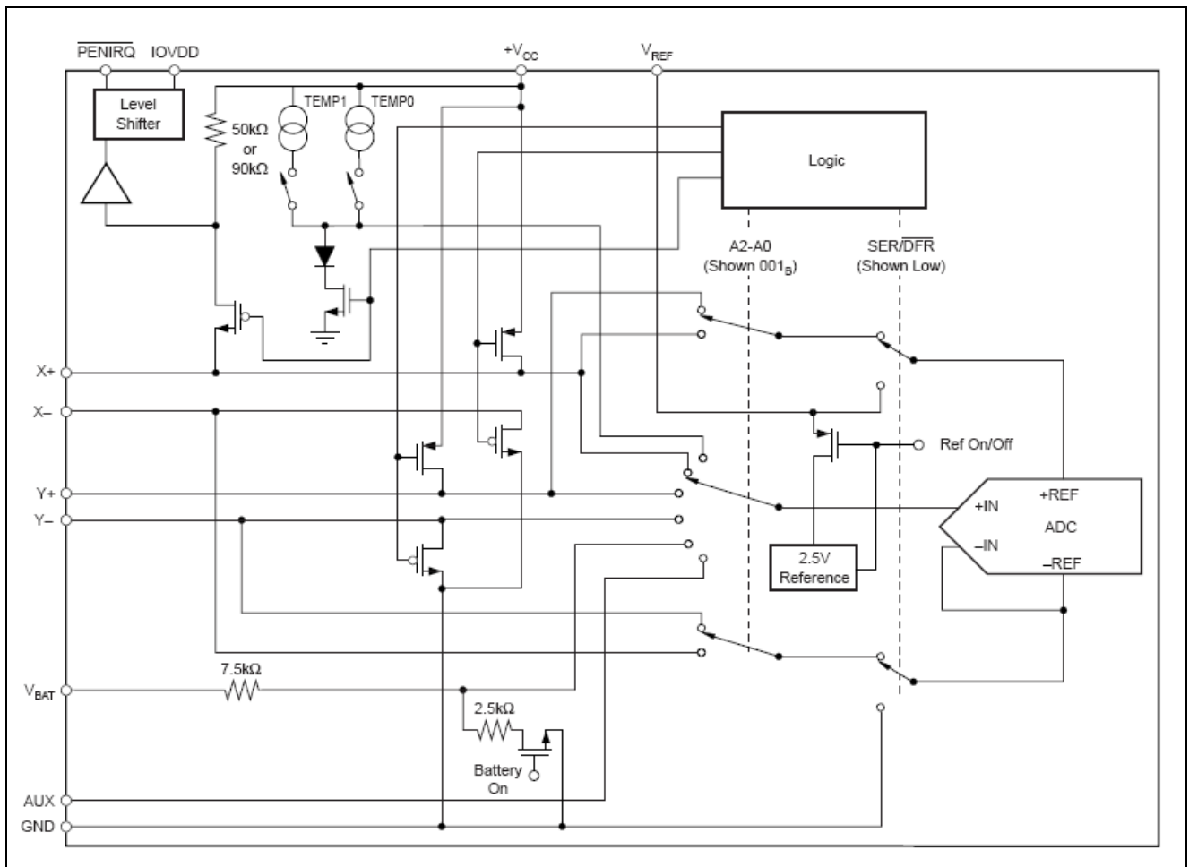
图 1 模拟输入
