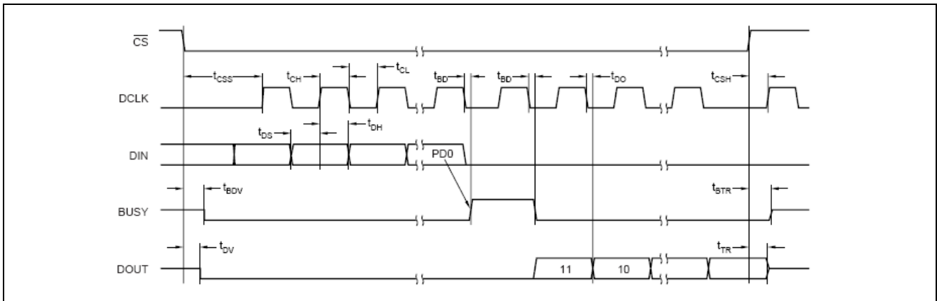
图 11 详细时序图
