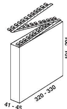
AMMO PACKAGING (mm)
