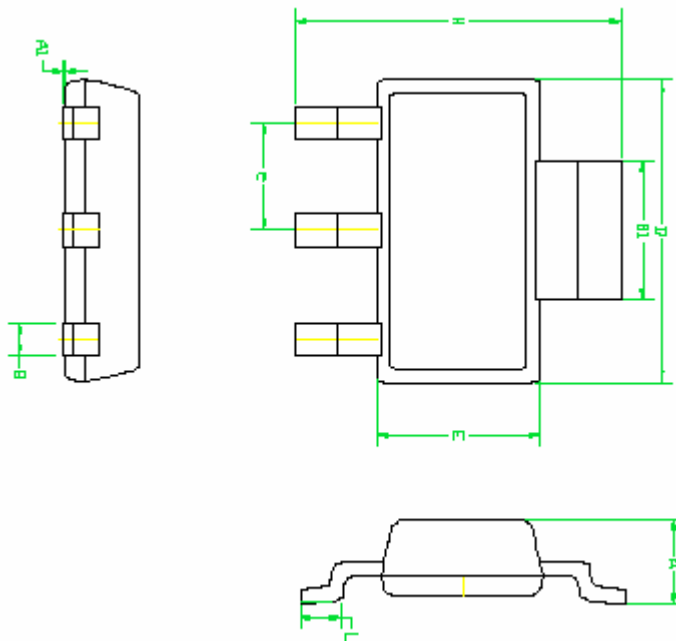
SOT223-3
