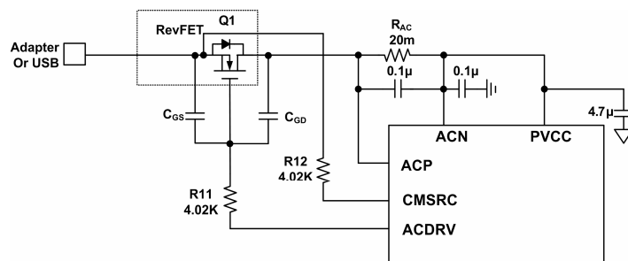
Figure 9. Input RevFET
