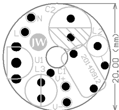
Figure1—Top Layer
