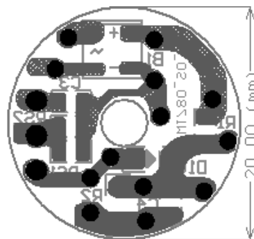
Figure2—Bottom Layer
