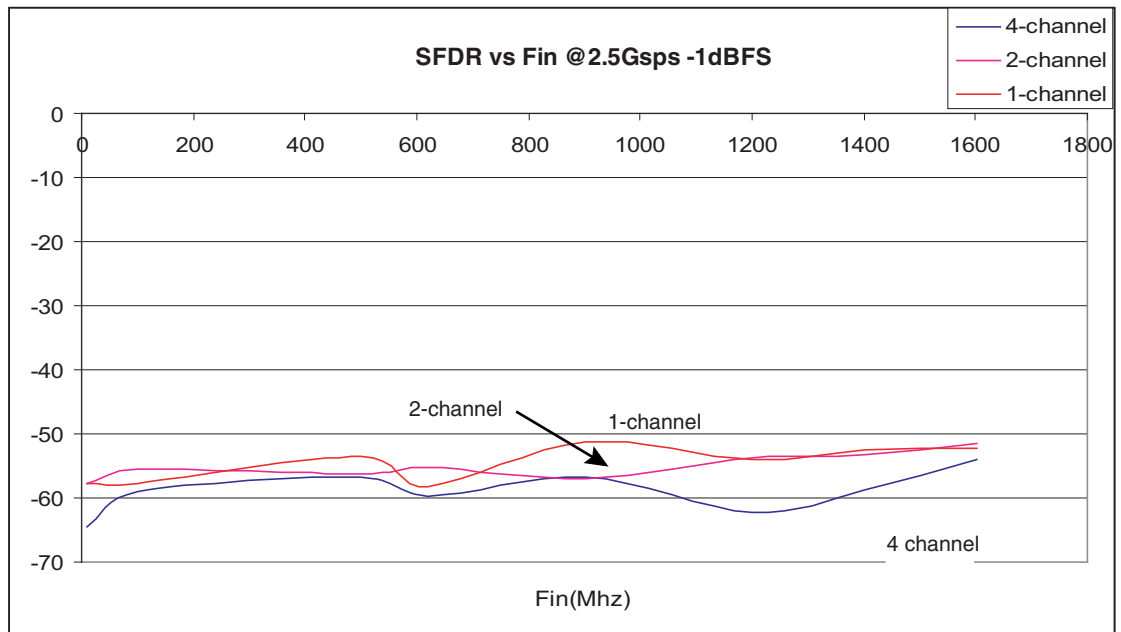
Figure 4-6. SFDR vs Fin
