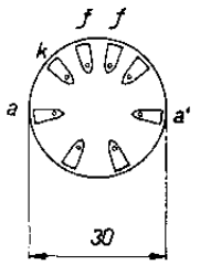
Connexions du culot du tube EZ 2.
