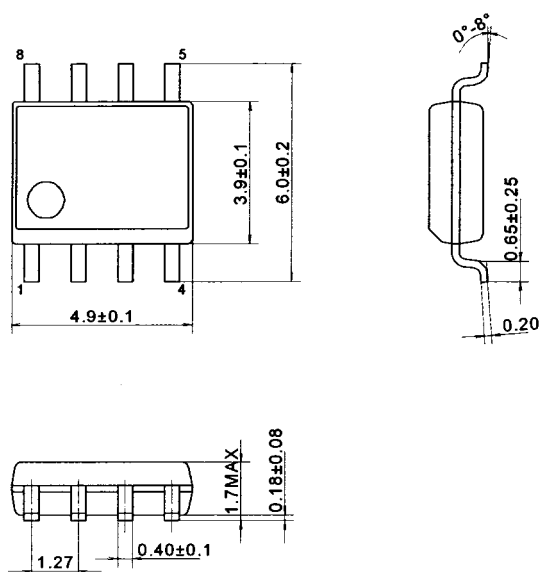
SOP-8 (FA5516N/FA5517N/FA5518N)
