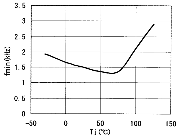
最低周波数( f_{min} ) vs. ジャンクション温度( T_j )
