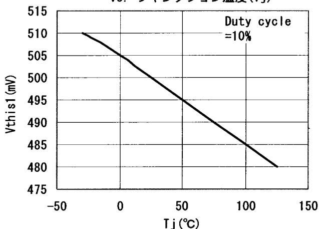
IS端子 最大入力スレッシュ電圧 ( V_{thi1} ) vs. ジャンクション温度 ( T_j )
