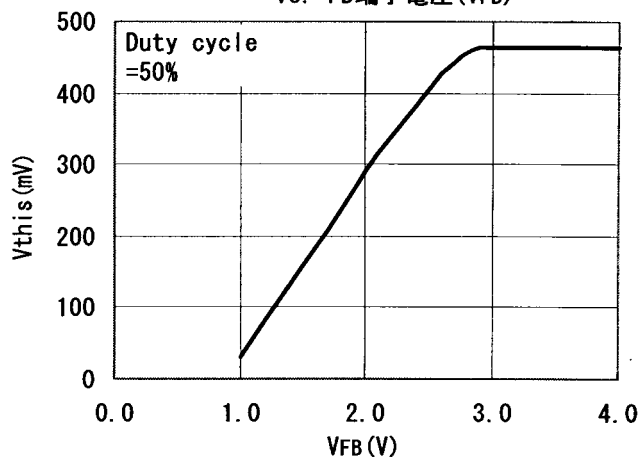
IS端子 入力スレッシュ電圧 ( V_{thi} ) vs. FB端子電圧 ( V_{FB} )
