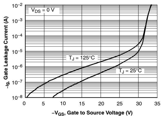
Figure 12. I_{gss} vs. V_{gss}
