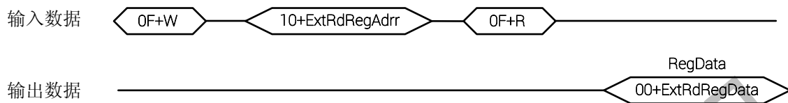
图 3-4 读扩展寄存器操作流
