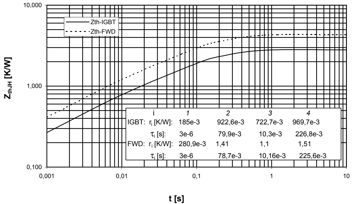
Transienter Wärmewiderstand Wechselr. Z_{thJH} = f(t) Transient thermal impedance Inverte
