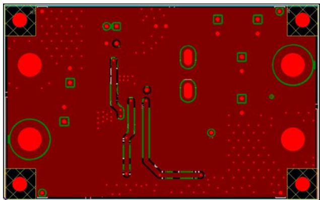
Figure 28. Bottom Layer
