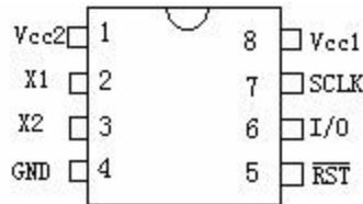
图 1 FS1002 引脚图
