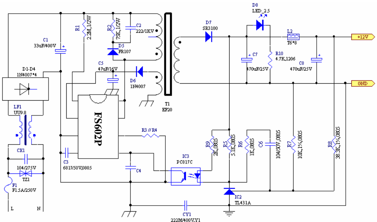
典型应用电路
