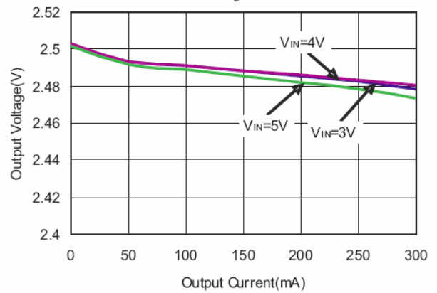
V_o = 2.5\text{V}
