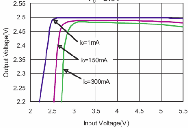
V_o = 2.5\text{V}
