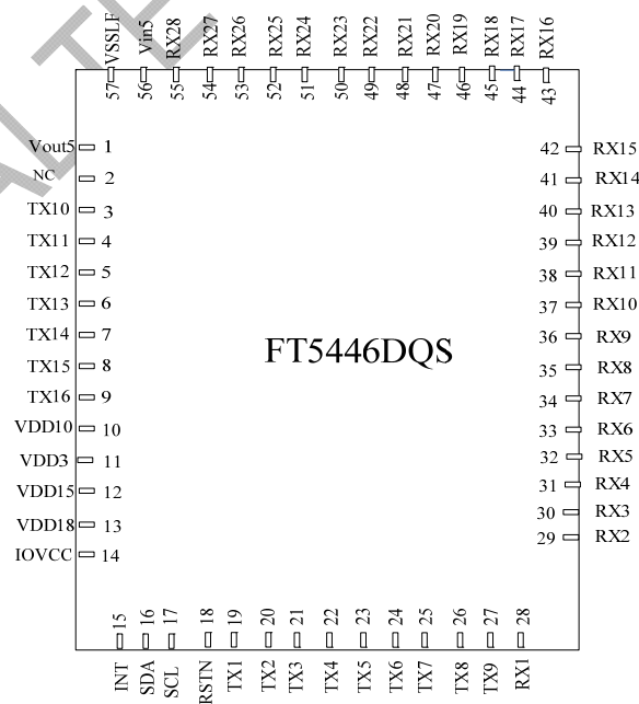
FT5446DQS Package Diagram
