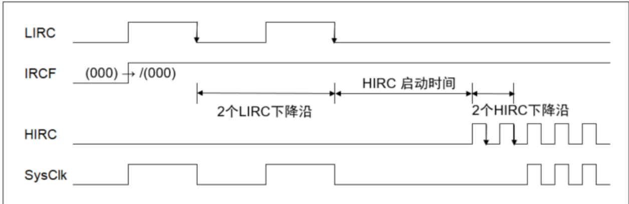
图 6-4 由 LIRC 切换到 HIRC 时序图 (同样的原则也适用于 EC, LIRC, HIRC 之间的切换)
